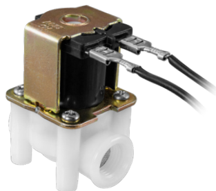
Рис. 2 – Клапан с выполненным подключением
